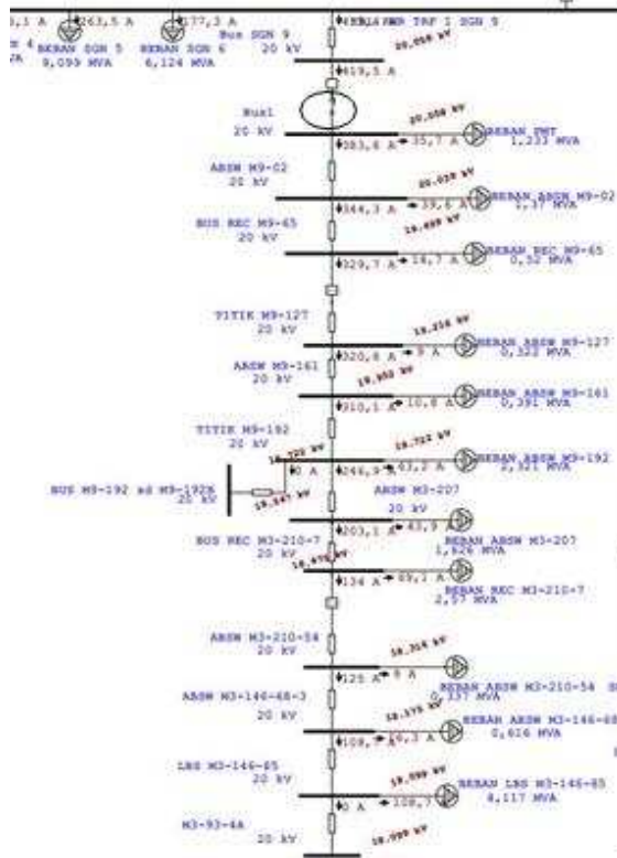
Gambar 4. SLD Simulasi Sebelum Kabelisasi
