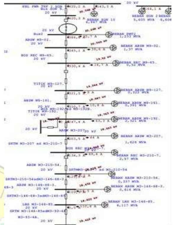
Gambar 5. SLD Simulasi Sesudah Kabelisasi
