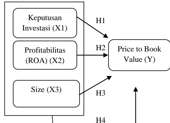
Gambar 1. Kerangka Pemikiran
