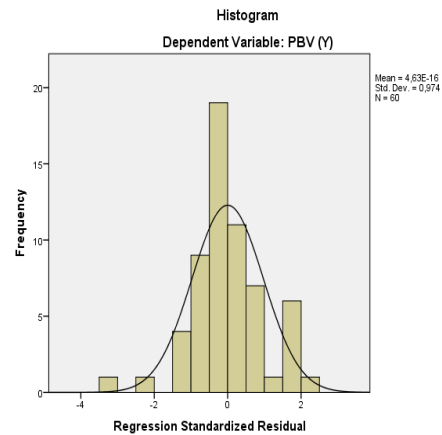
Gambar 2. Grafik Histogram
